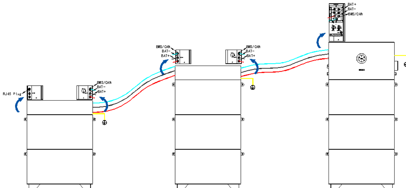
Figure 5.30. Collegamento di otto batterie in tre stack
