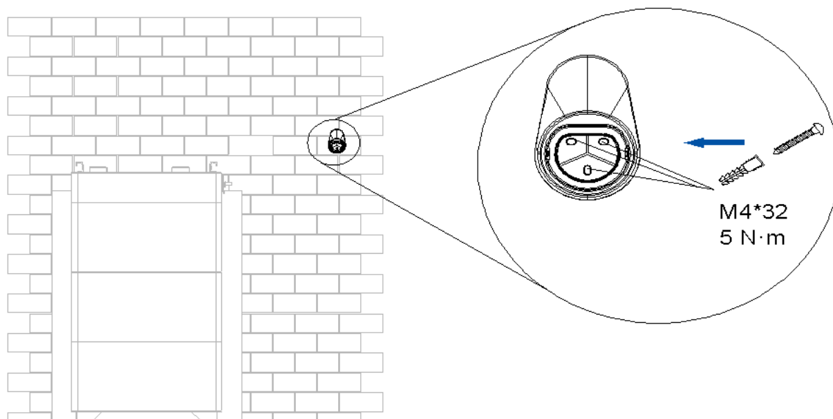
Figure 4.24. Installazione della custodia del cavo del caricabatterie
