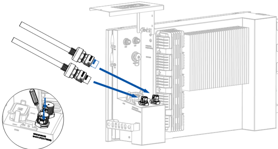
Figure 5.12. Collegamento dei cavi di rete e di carico di backup
