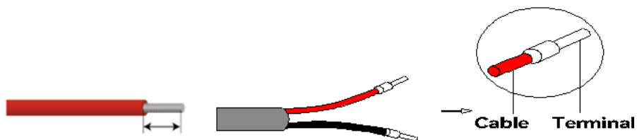
Figure 5.14. Installazione dei terminali a crimpare isolati alle estremità del cavo
