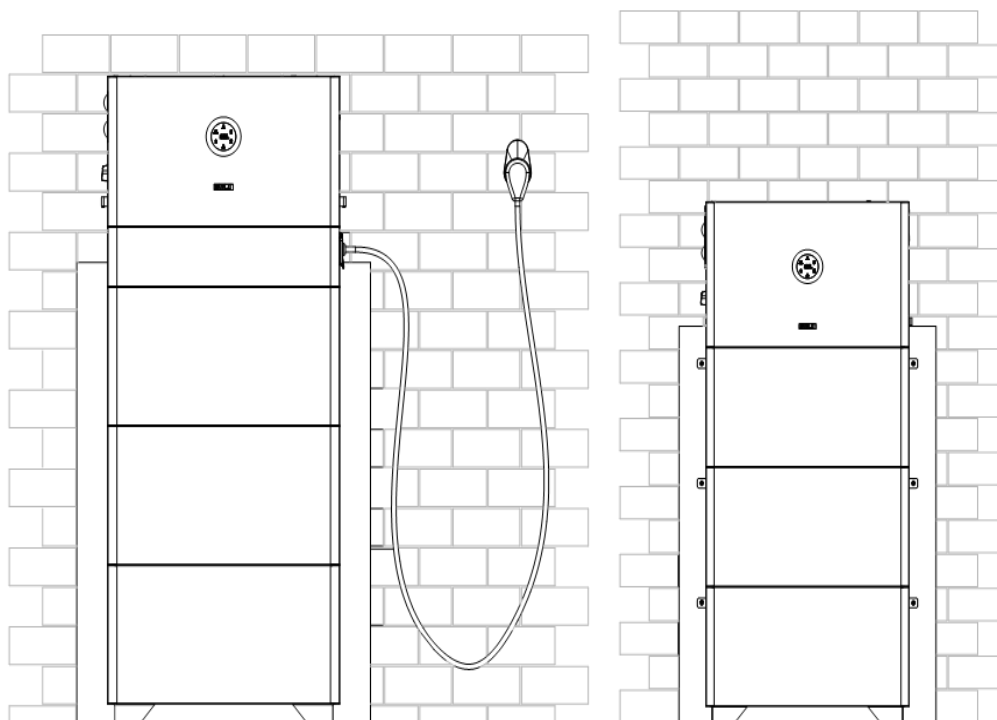
Figure 4.27. Vista completa di una singola pila
