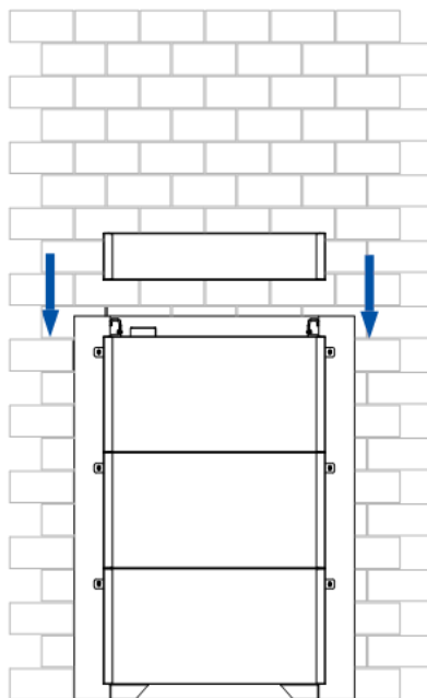
Figure 4.44. Installazione di una scatola di giunzione della batteria
