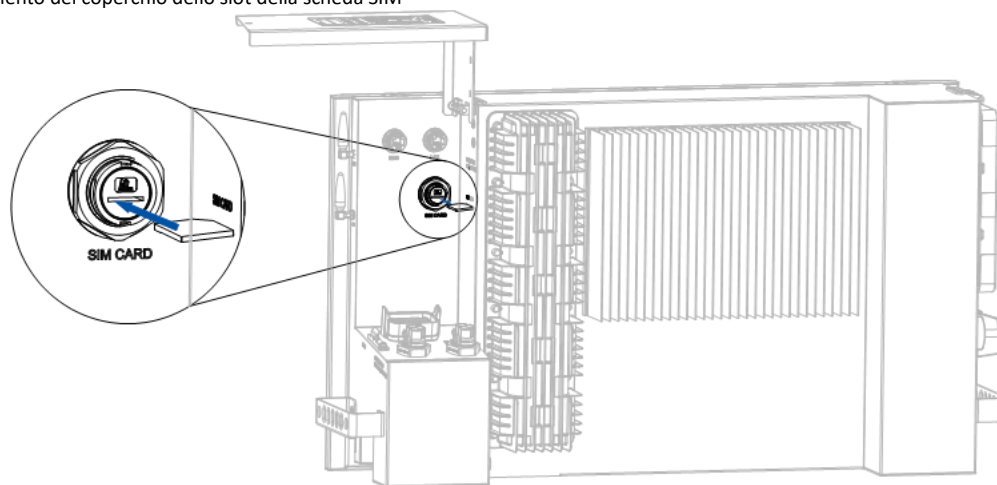
Figure 5.6. Inserimento della scheda SIM
