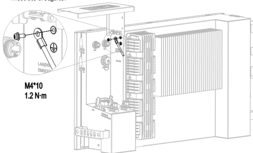
Figure 5.4. Collegamento del cavo di messa a terra aggiuntivo
