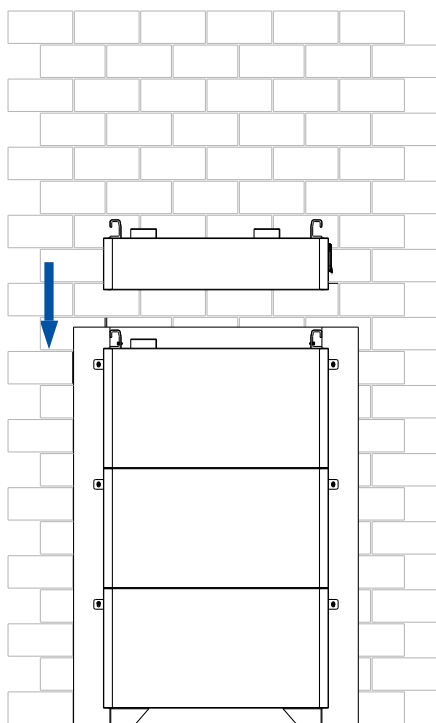
Figure 4.12. Installazione del caricabatterie
