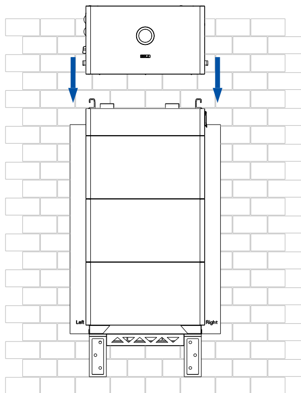
Figure 4.42. Installazione dell'inverter
