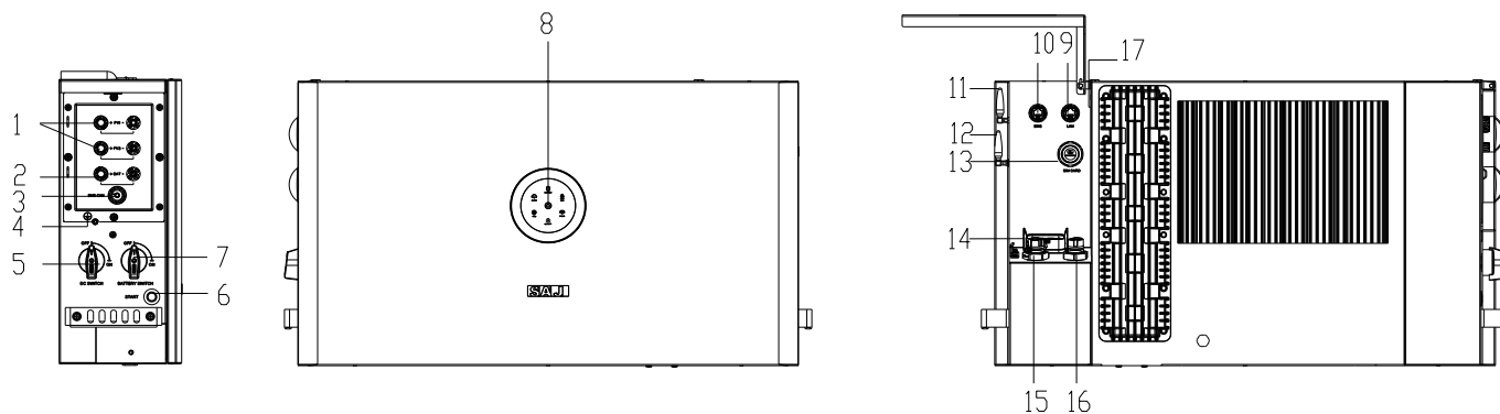
Figure 2.7. Porte, interruttori e LED sull'inverter HS3
