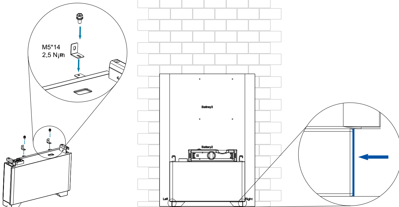
Figure 4.18. Installazione della batteria con la base
