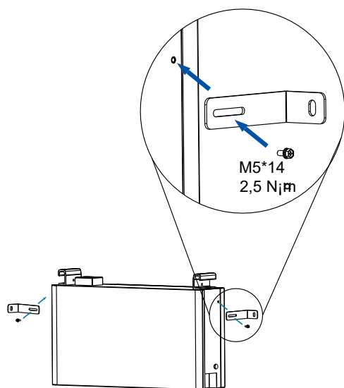
Figure 4.9. Installazione della seconda batteria
