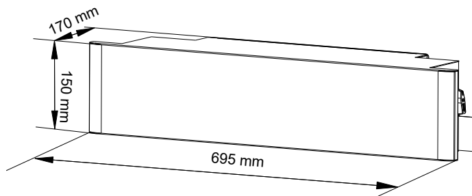
Figure 2.5. Dimensioni della scatola di giunzione per batterie BC3
