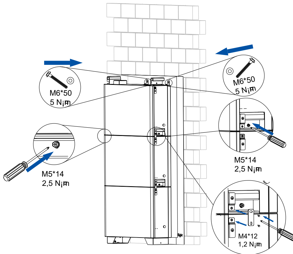
Figure 4.22. Installazione della terza batteria
