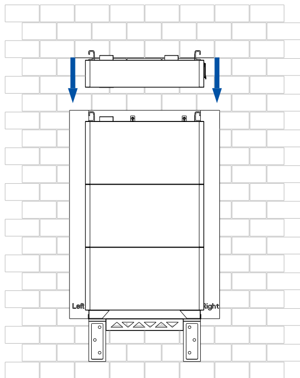
Figure 4.39. Installazione del caricatore
