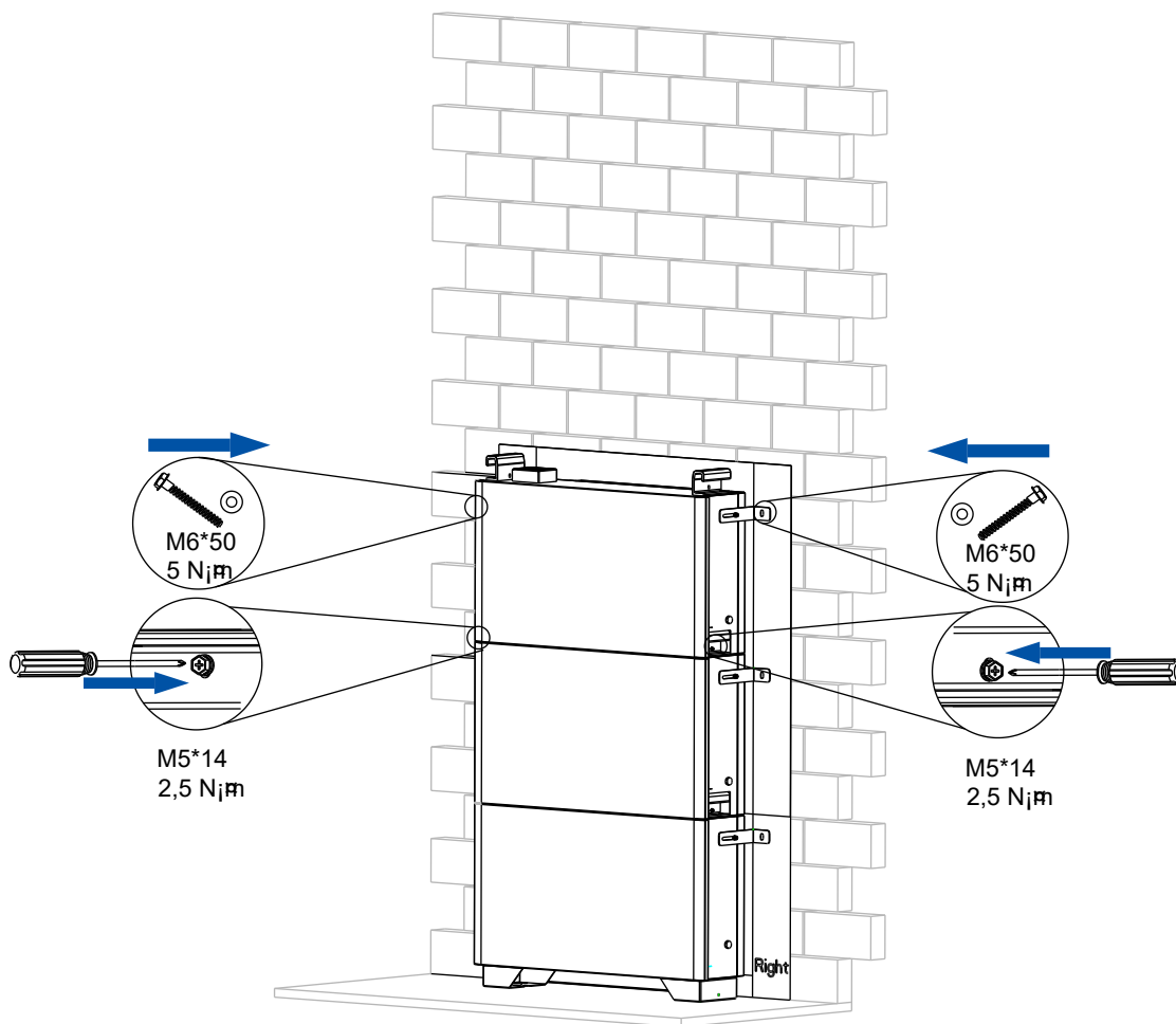
Figure 4.11. Installazione della terza batteria
