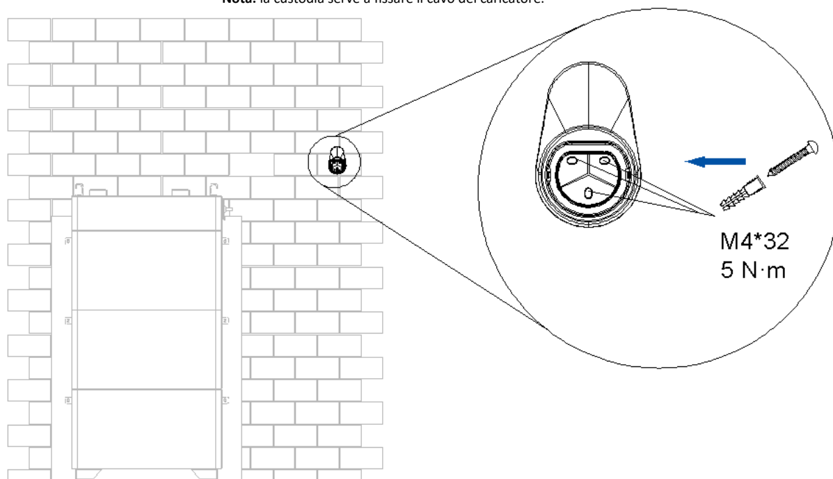
Figure 4.13. Installazione della custodia del cavo del caricabatterie
