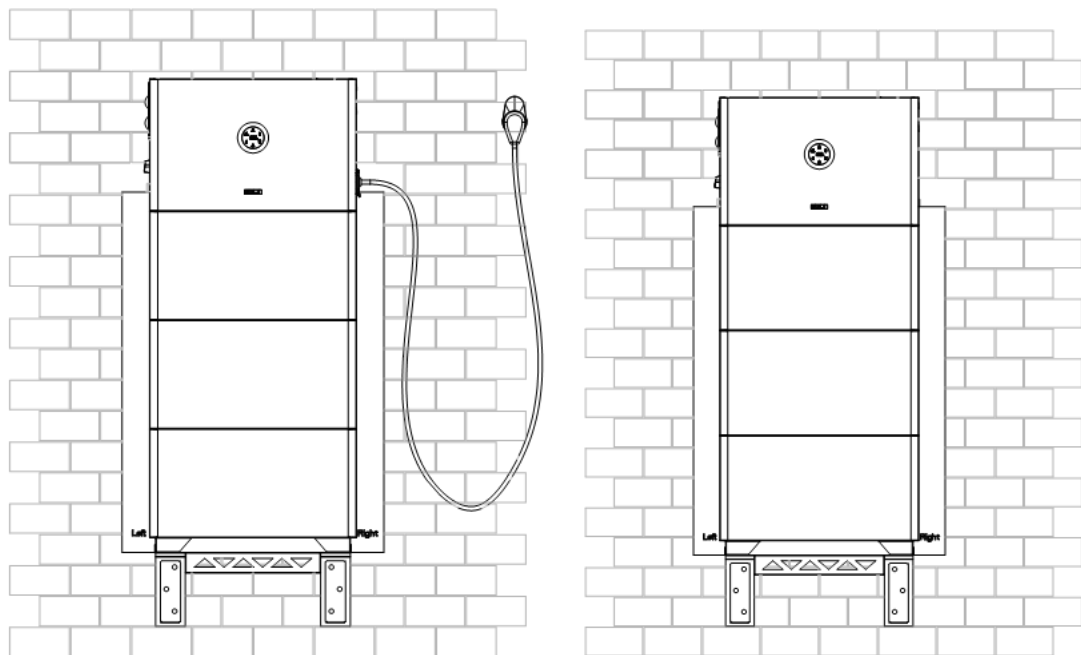
Figure 4.43. Vista finale di una singola pila
