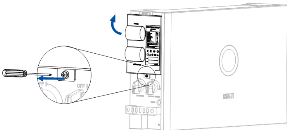
Figure 5.21. Apertura del coperchio lato CC
